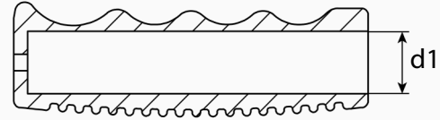
KESİT A-A
